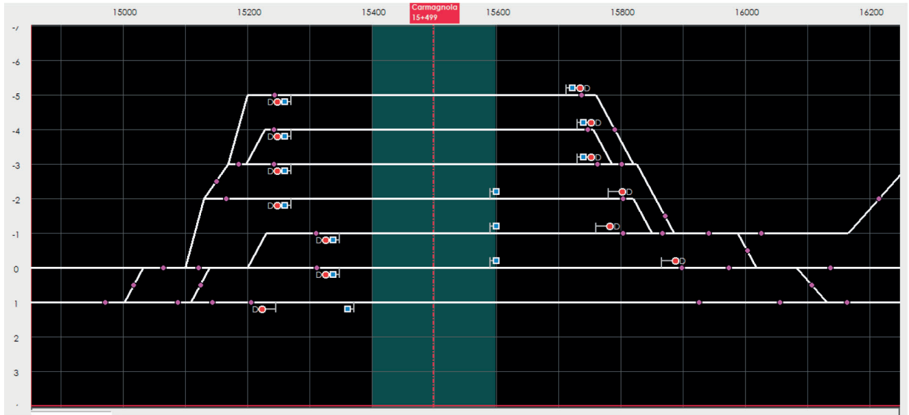
Figura 8 – Editor del pacchetto di calcolo SASTRE. In figura la stazione di Carmagnola. Figure 8 – Editor of the SASTRE calculation package. The Carmagnola station is shown in the figure.
