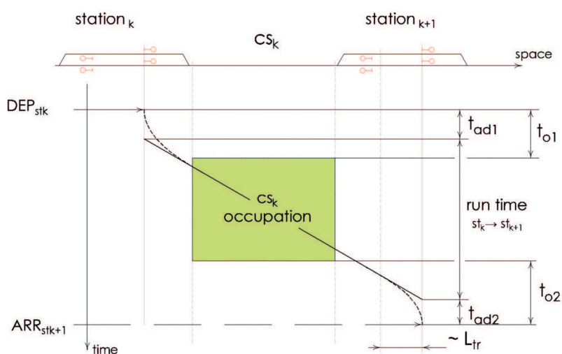
Fig. 2 - Parametri impiegati nel modello mesoscopico.
