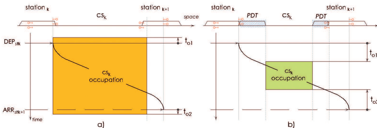
Fig. 4 - Tempo di occupazione di una CS nel caso di assenza (a) e presenza (b) di doppio binario parziale (PDT, partial double track).
